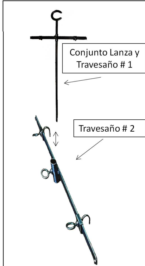
PASO 2: Unir conjunto con Travesaño # 2
